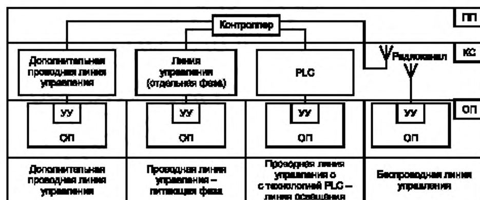
Рисунок 8 — Схема комбинированных каналов связи
