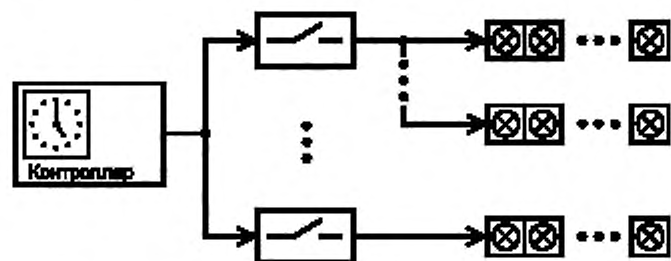
Рисунок 1 — Автоматический режим переключения с учетом времени суток
